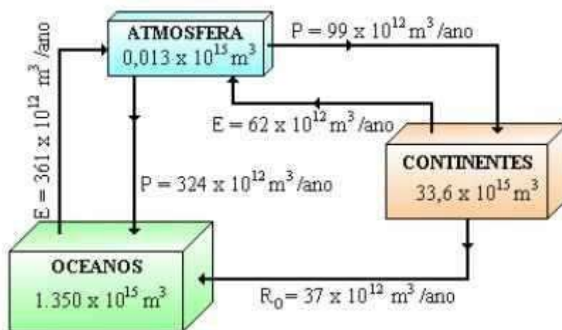
Figura 2 - Volume armazenado d'água nos oceanos, nos continentes e na atmosfera e precipitação pluvial (P), evaporação (E) e "runoff" (R 0 ). Fonte: Peixoto e Oort (1992)
