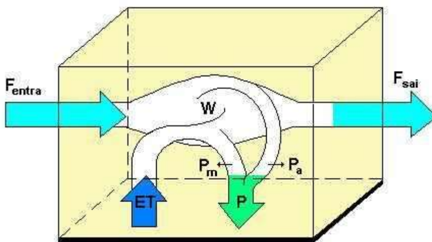
Figura 3 - Reciclagem de vapor d'água na atmosfera.
